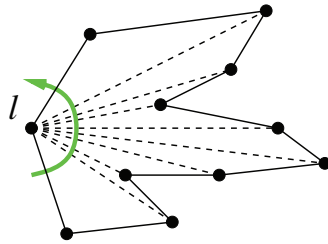
Abb.: Durch die radiale Sortierung betrachtet der Algorithmus die Punkte (implizit) entlang eines simplen Polygons
